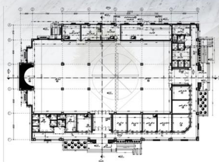
پلان تراز 0.45
