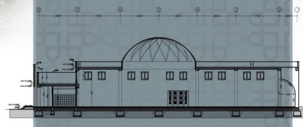
مقطع A.A
