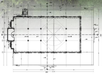
پلان تراز 4.45
